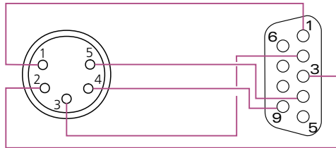
VCA500 Fiche XLR femelle 5 points
